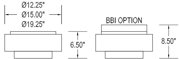
WHL diffuser
