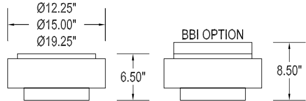
WHL diffuser
